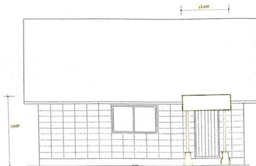
前面図 1/50
