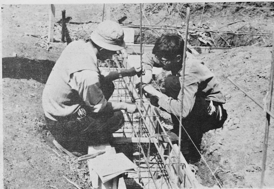
5月大学創立60周年記念日 青写真と首っぴきで鉄骨組みを行う
