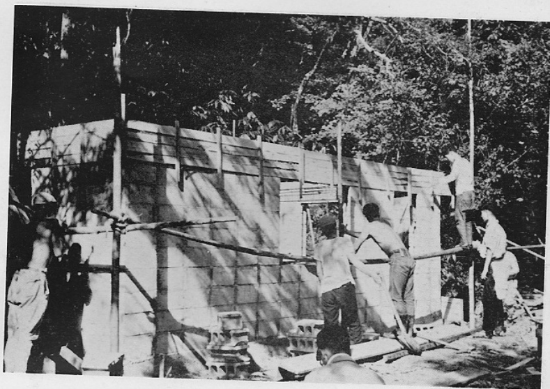
10月 難関の臥梁打ちはやむなく大工の手を借りた
